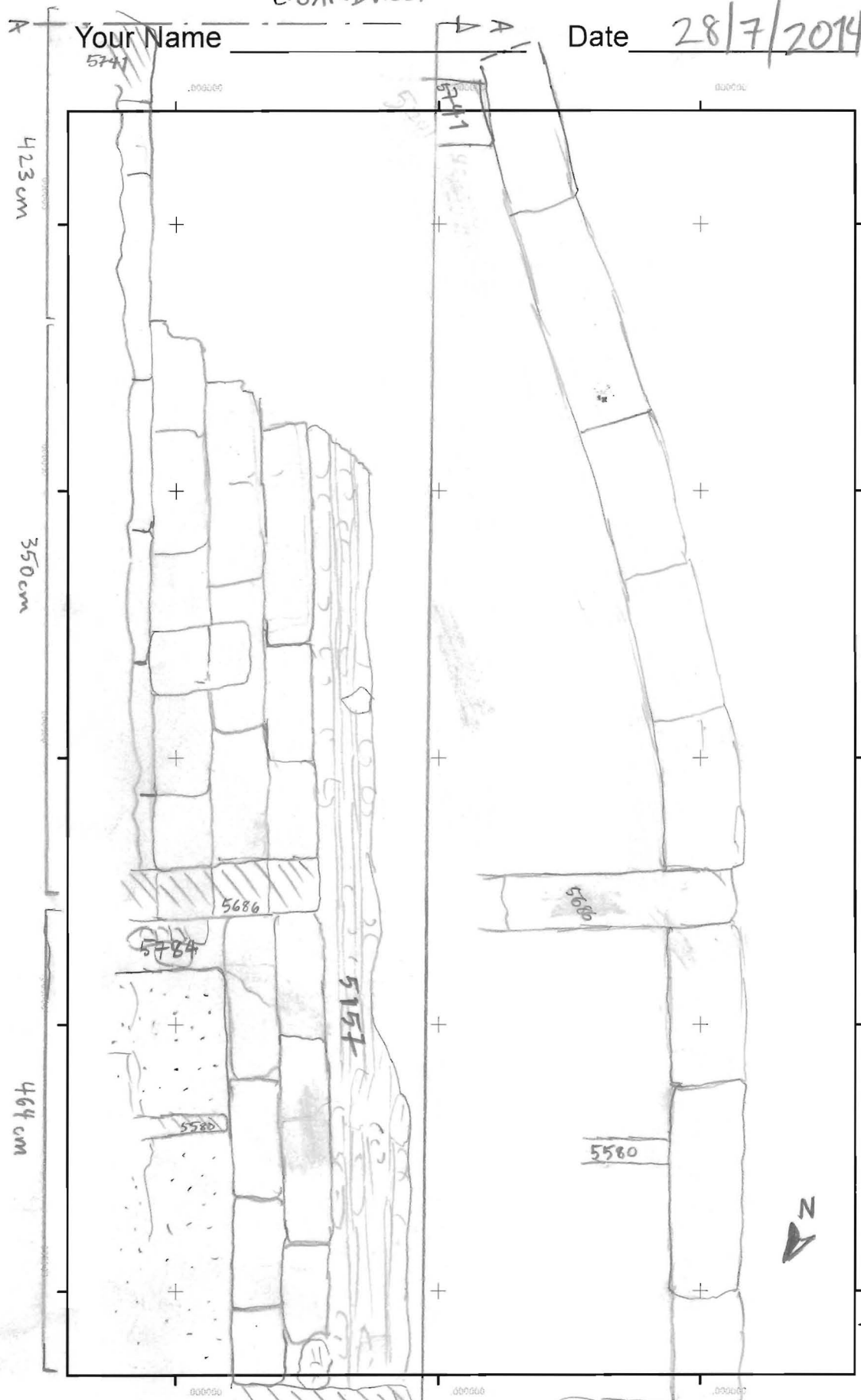
ELEVATION
